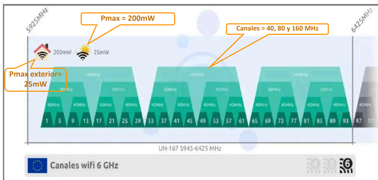
Canales WiFi 6E en 6 GHz en España, con los canales ilegales en Europa a partir del 97
