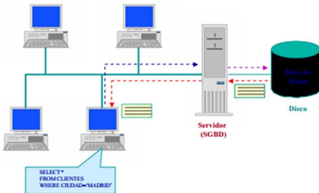
Figura 5.4: Arquitectura De Bases de Datos Cliente/Servidor
