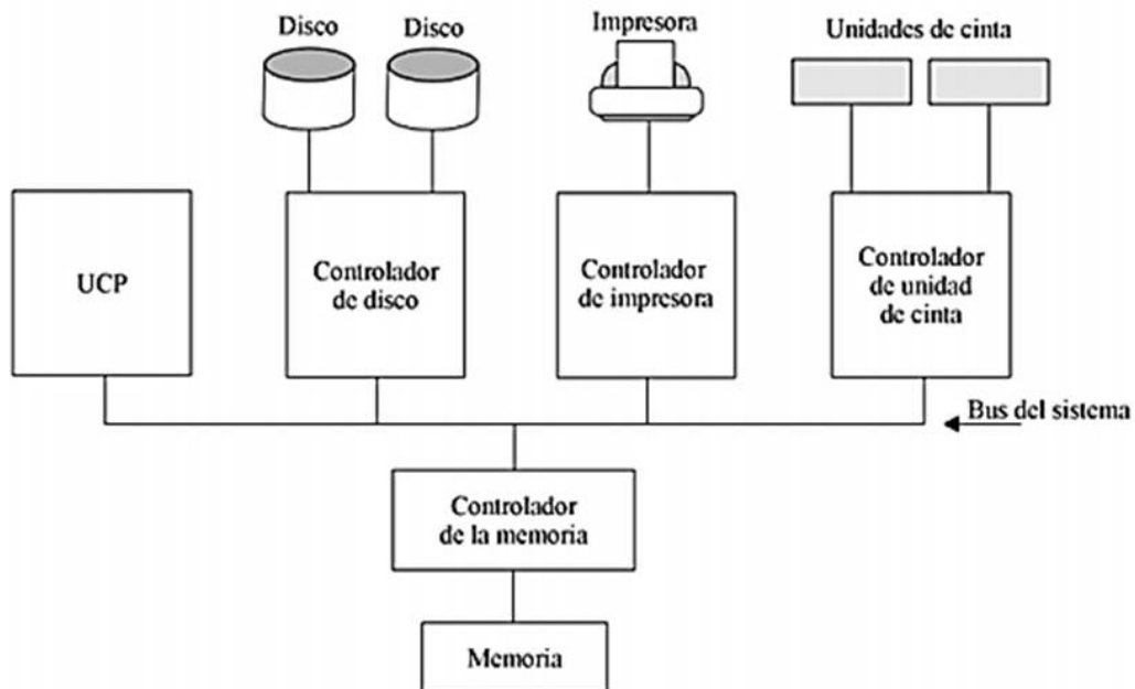
Figura 5.3: Arquitectura Centralizada
